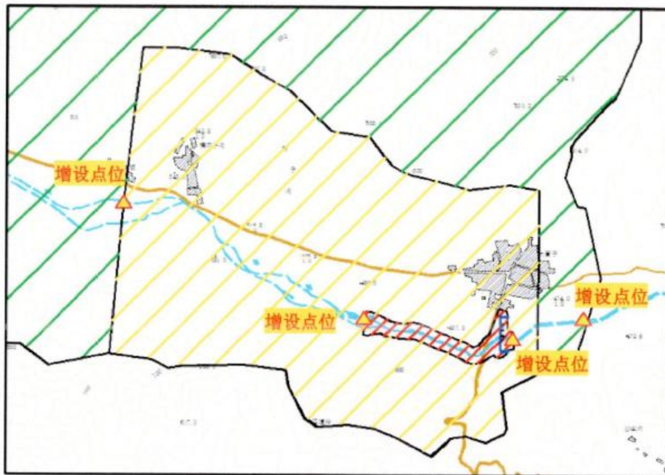
附图6大营子集水廊道监日常测点位示意图
