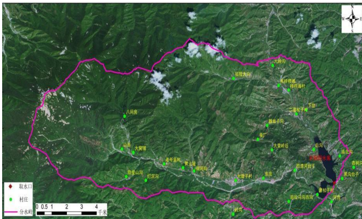
图 3-2 水库流域范围内居民村庄分布图
