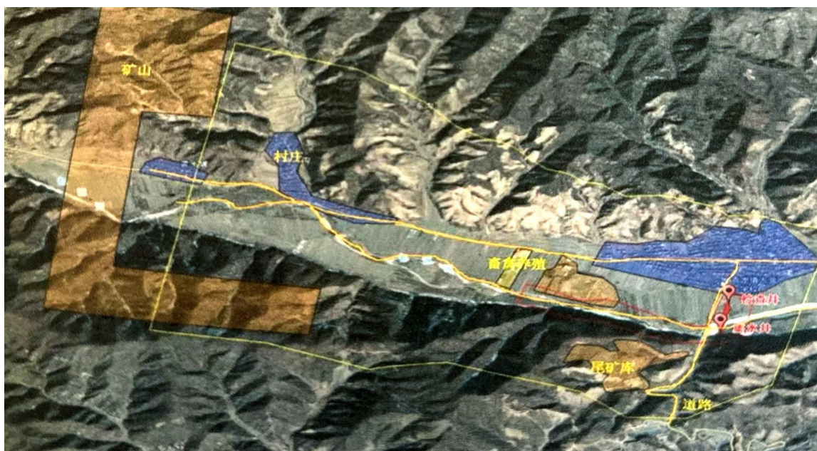
图 3-4 大营子水源地一、二级保护区主要污染源分布图
