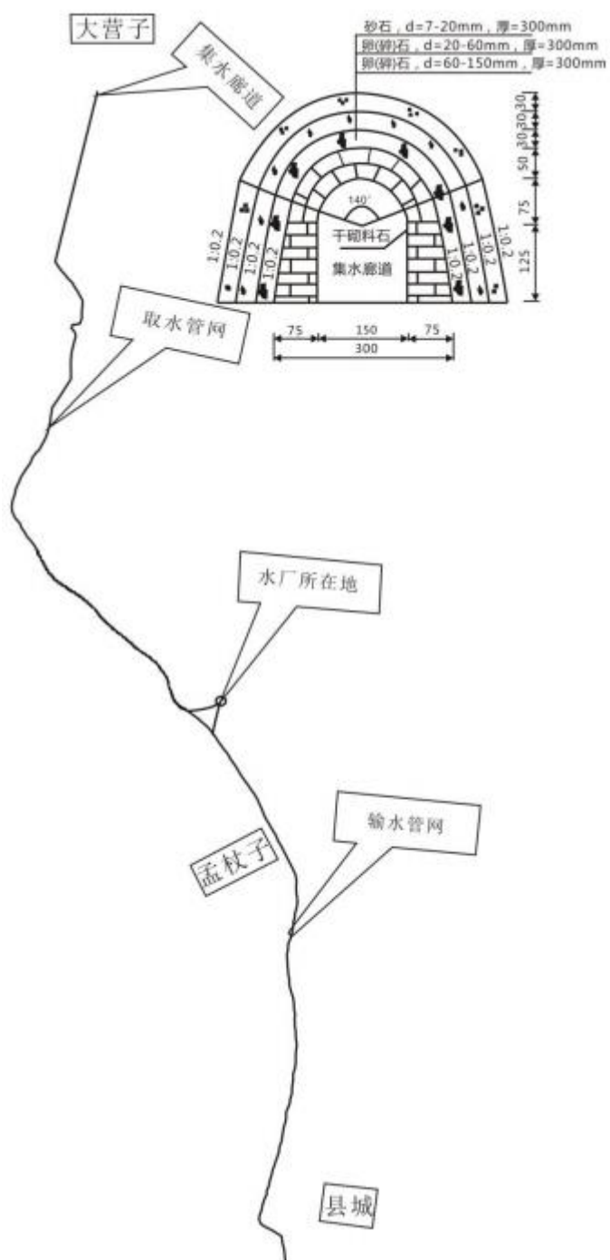
图 2-3 集水廊道横断面图和供水工程路线图
