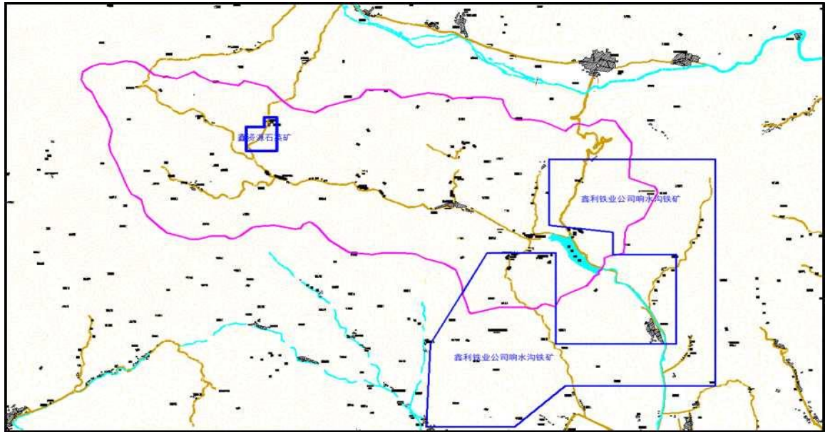
图 3-5 水库流域分水岭范围内矿山分布情况
